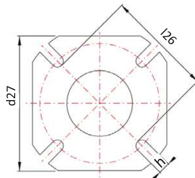
Подвійне ущільнення R-TSSC-A05
