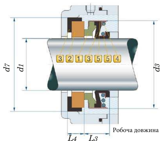
Торцеве механічне ущільнення R-BT-AR
