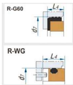
Тип контркіля
