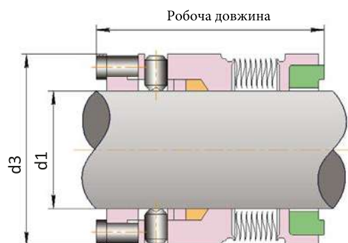
Механічне торцеве ущільнення R-609
