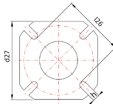
Двойное уплотнение R-TSSC-A05
