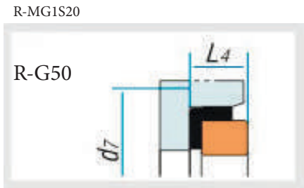
Тип контркольца
