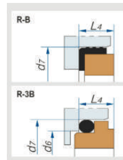
Тип контркольца
