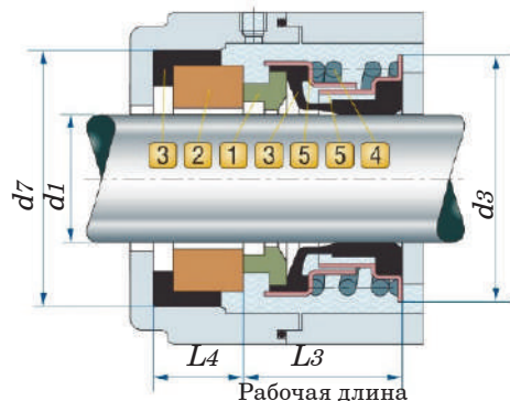
Механическое торцевое уплотнение R-6/16
