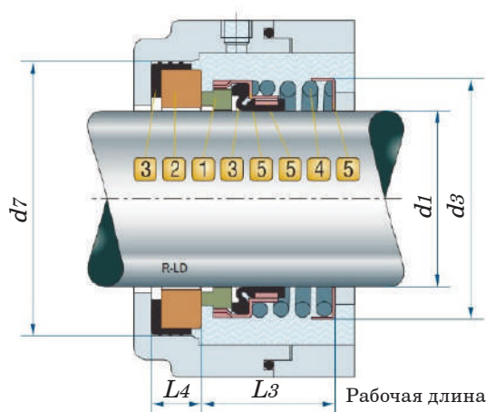
Торцевое механическое уплотнение R-560A
