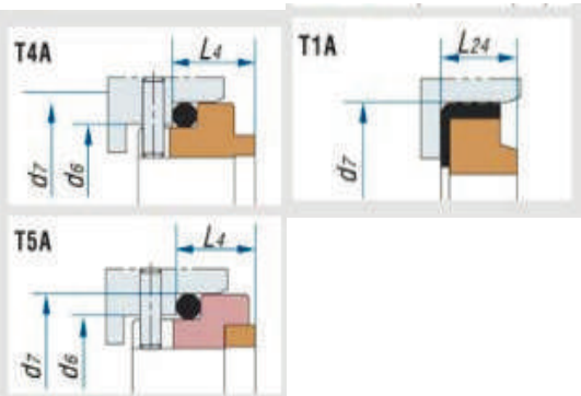
Тип контркольца
