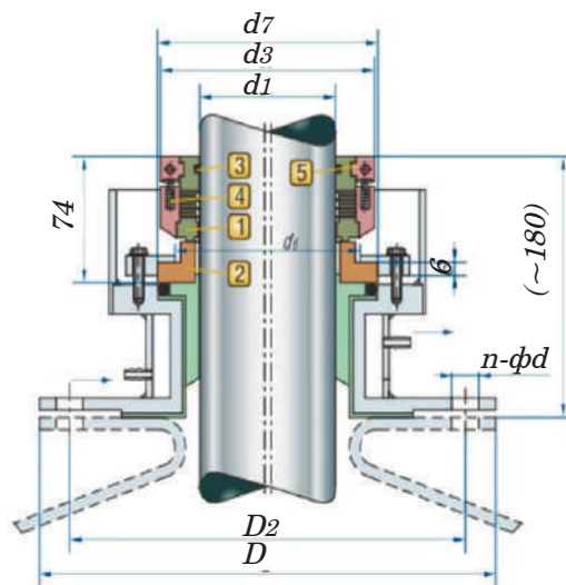
Одинарное торцевое уплотнение R-HG212
